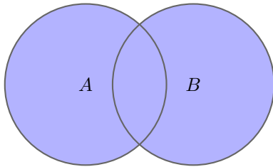
A \cup B Vereinigung
