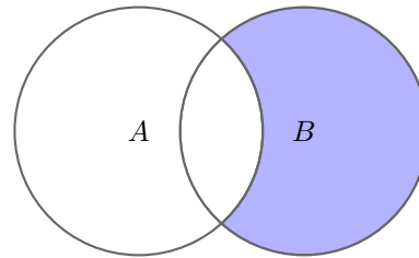
B \setminus A
