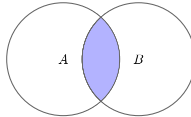
A \cap B Schnitt
